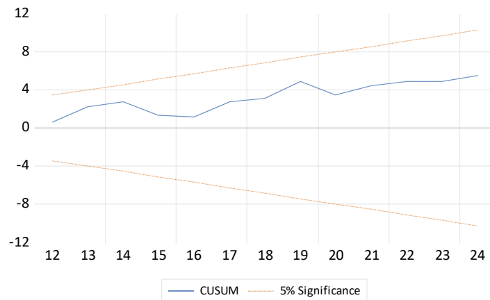
ภาพที่ 2 ค่า CUSUM test ของสมการอัตราดอกเบี้ยโตทางเศรษฐกิจ ARDL (4,4,3)
