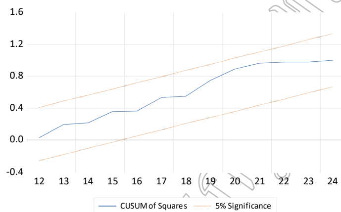
ภาพที่ 3 ค่า CUSUM squares test ของสมการอัตราดอกเบี้ยโตทางเศรษฐกิจ ARDL (4,4,3)
