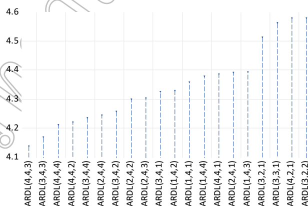
ภาพที่ 2 การเลือกแบบจำลองที่เหมาะสมโดยใช้เกณฑ์ AIC
